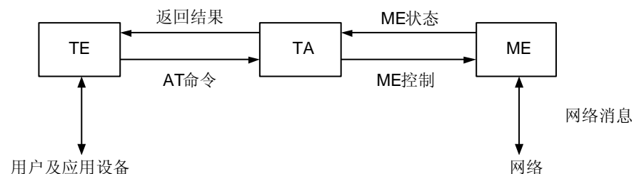
图1-1 系统结构图
