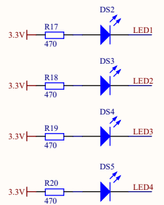
四轴指示灯
