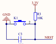
复位电路
