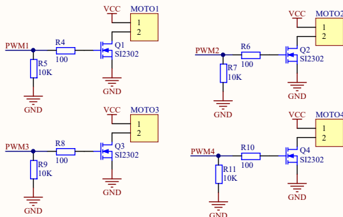
电机
