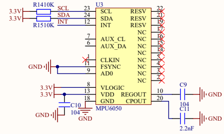
陀螺仪MPU6050
