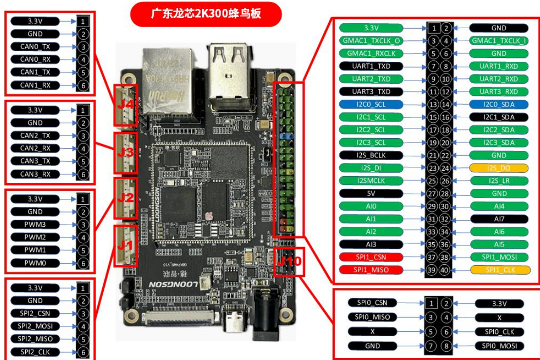
广东龙芯 2K300 蜂鸟板扩展接口图
