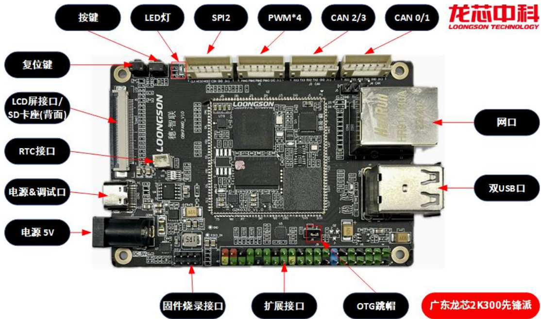
广东龙芯 2K300 蜂鸟板接口图
